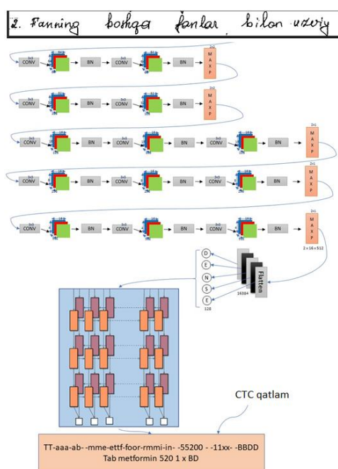
5-rasm. CNN+LSTM+CTC model arxitekturası
