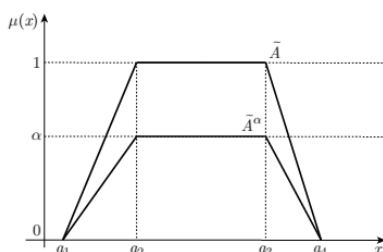
1-рasm. Ишончилиликни кўпайтиргандан кейинги Z-сон
