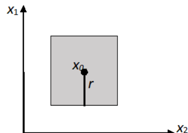
Рис. 3.2a Шар радиуса r в R^n в супремальной метрике
