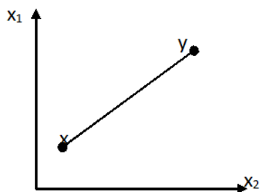
Рис.1.16 Отрезок между двумя точками в R^n
