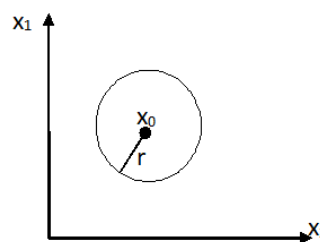
Рис. 1а Шар радиуса r с центром в точке x_0 в R^n
