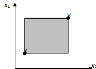
Рис.2.2б Отрезок между двумя точками в R^n в манхеттенской метрике
