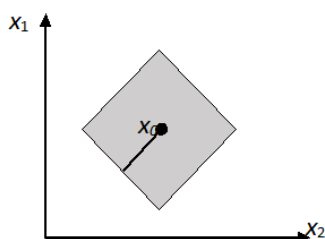
Рис.2.2a Шар радиуса r в R^n в манхеттенской метрике
