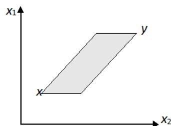
Рис.3.6 Отрезок между двумя точками в R^n в супремальной метрике
